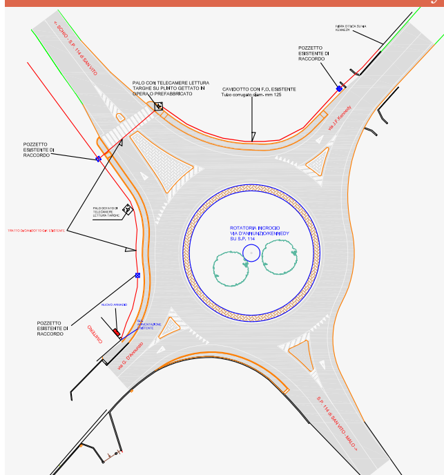
Rotatoria incrocio Via D'Annunzio - Via Kennedy
