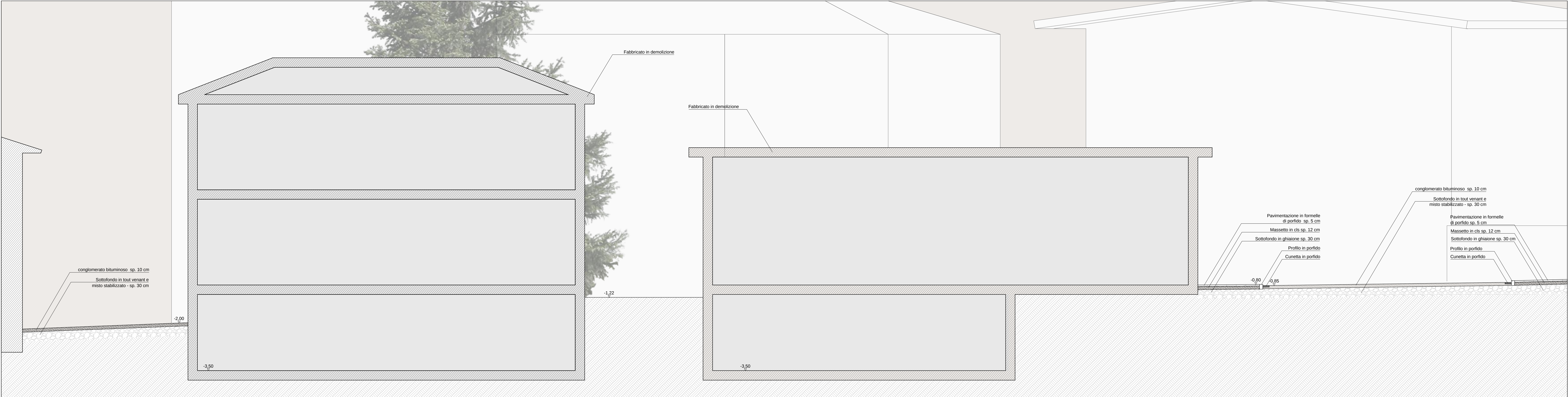
STATO DI FATTO | SEZIONE B-B | SCALA 1:50
