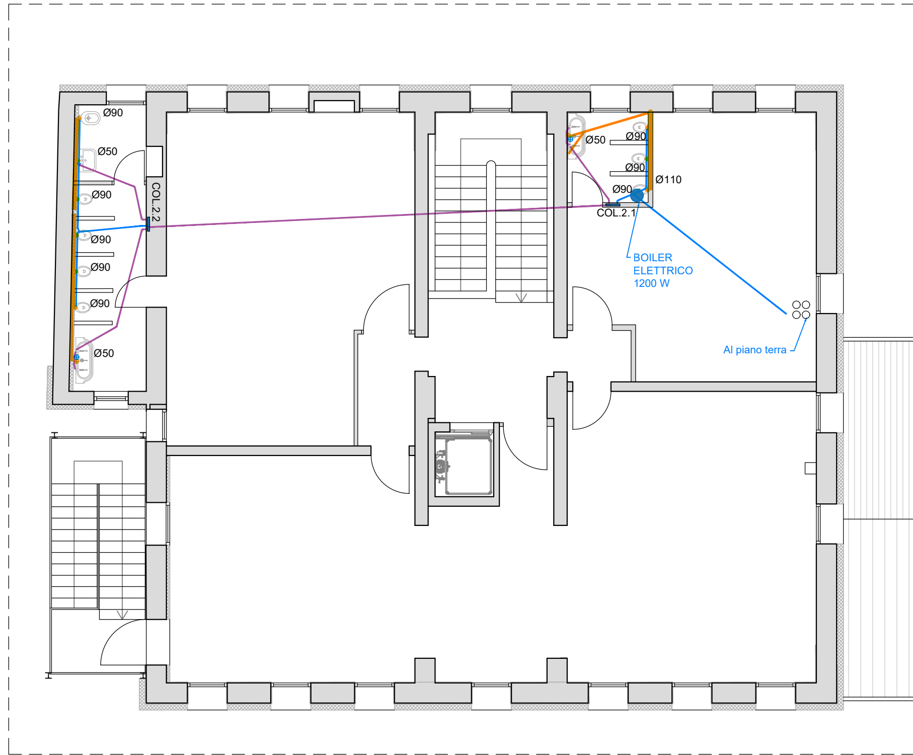
PIANTA PIANO SECONDO SCALA 1:100
