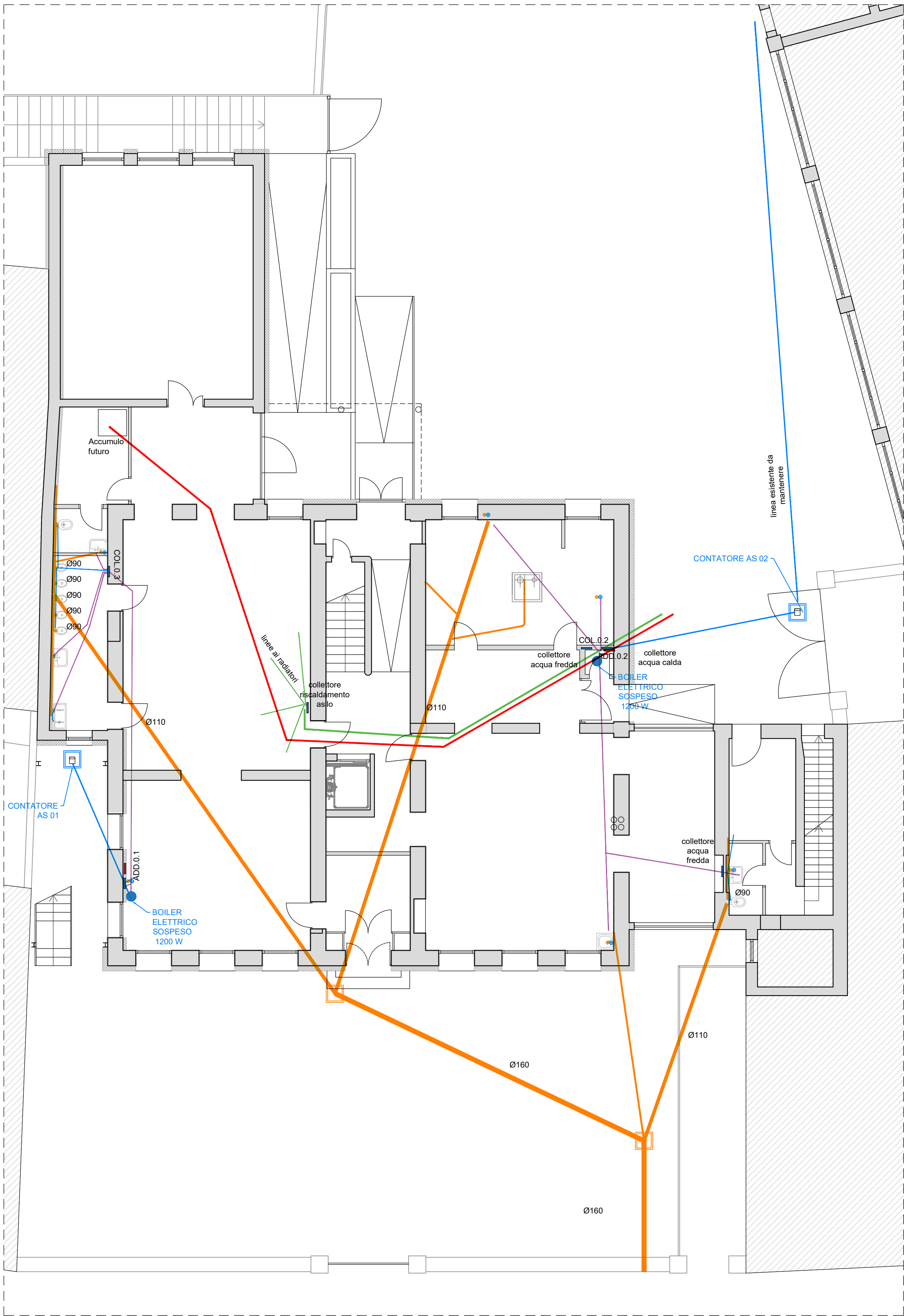
PIANTA PIANO TERRA SCALA 1:100
